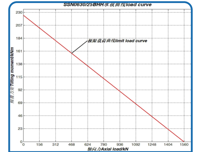
序号 8、SSN0630/25BHH 承载曲线
