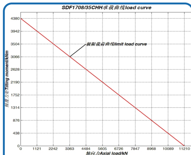
序号 11、SDF1708/35CHH 承载曲线
