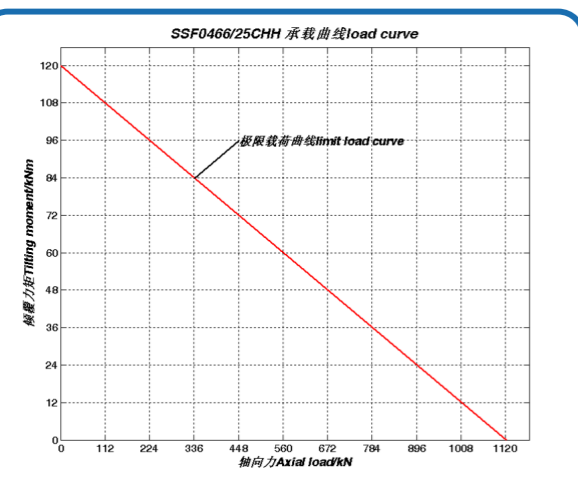
序号 1、SSF0466/25CHH 承载曲线
