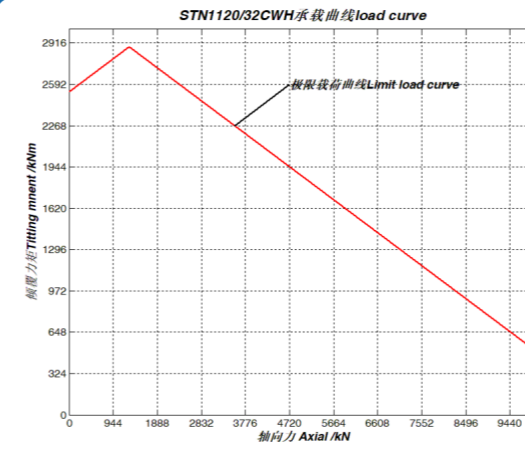
序号 7、STN1120/32CWH 承载曲线
