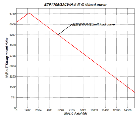
序号 1、STF1705/32CWH 承载曲线
