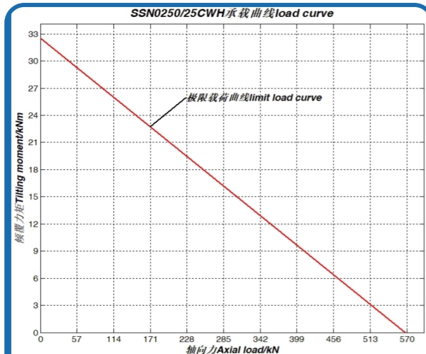
序号 1、SSN0250/25CWH 承载曲线
