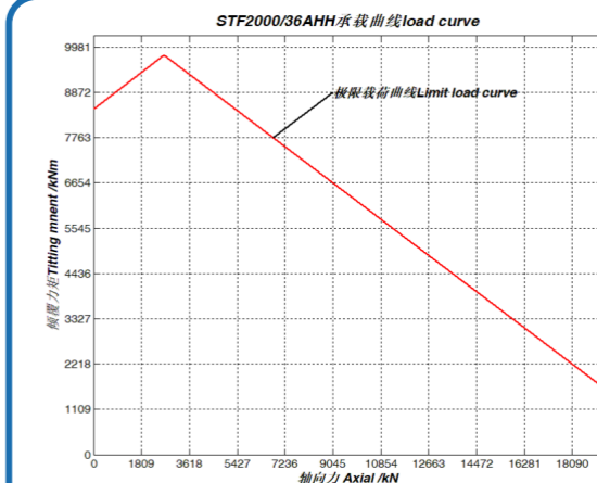
序号 4、STF2000/36AHH 承载曲线
