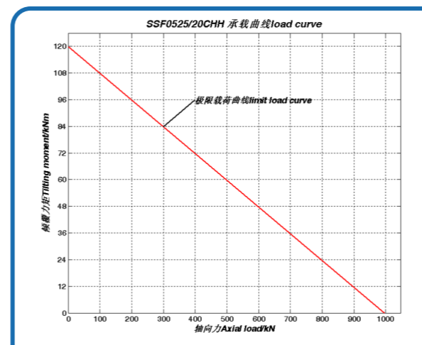
序号 3、SSF0525/20CHH 承载曲线
