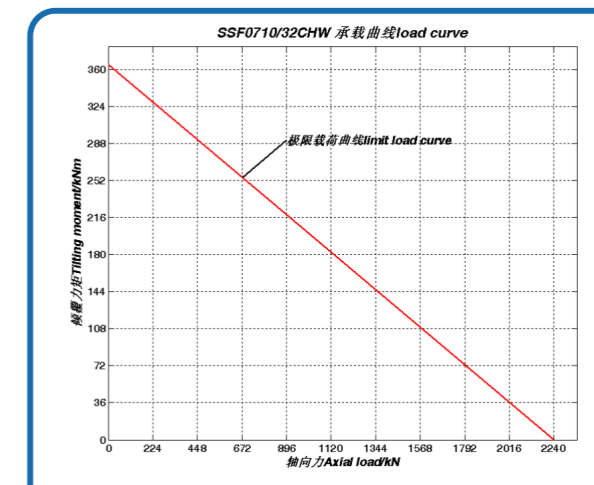
序号 6、SSF0710/32CHW 承载曲线
