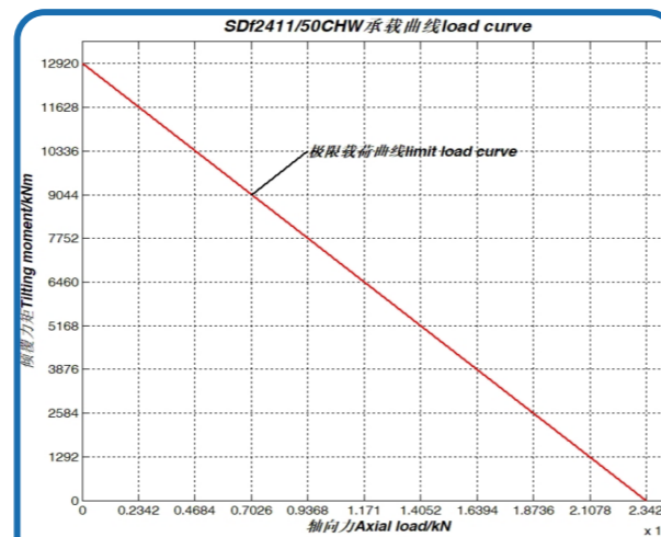
序号 22、SDF2411/50CHW 承载曲线
