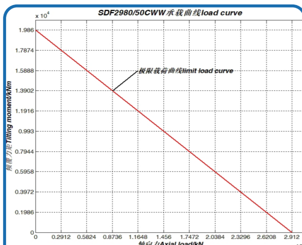
序号 25、SDF2980/50CWW 承载曲线
