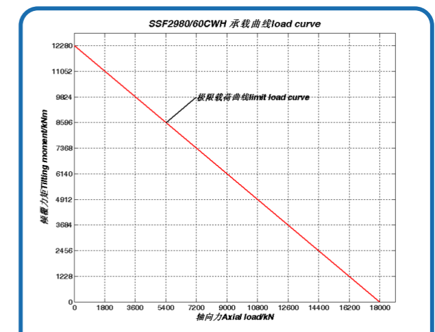
序号 68、SSF2980/60CWH 承载曲线
