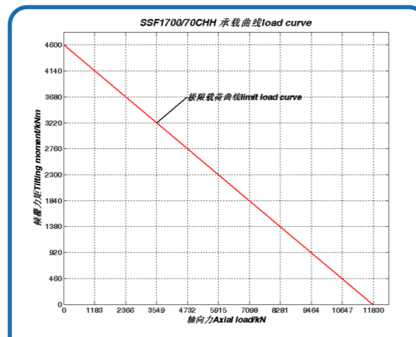
序号 60、SSF1700/70CHH 承载曲线
