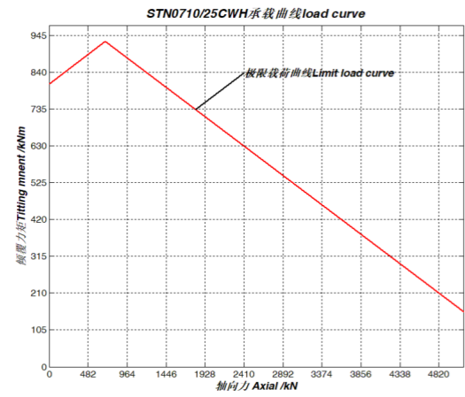
序号 1、STN0710/25CWH 承载曲线
