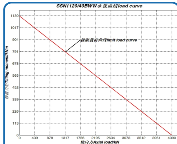
序号 14、SSN1120/40BWW 承载曲线
