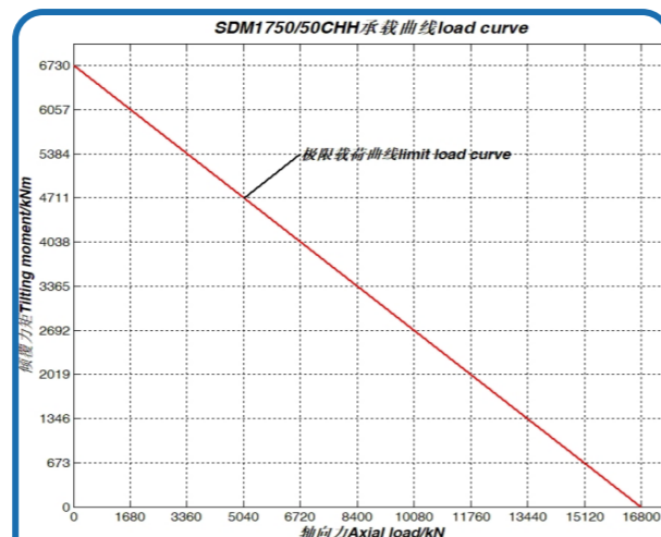
序号 12、SDM1750/50CHH 承载曲线
