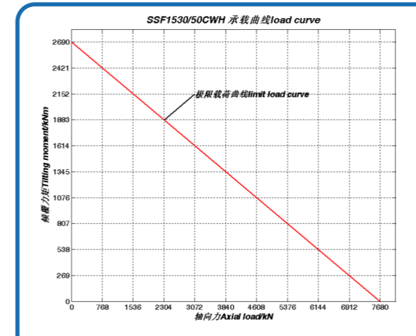
序号 51、SSF1530/50CWH 承载曲线
