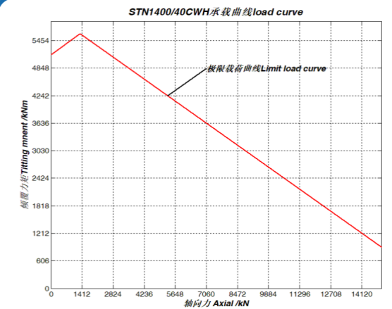
序号 10、STN1400/40CWH 承载曲线
