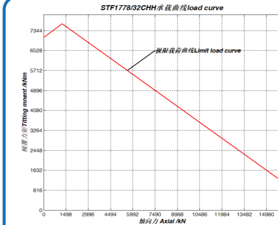
序号 2、STF1778/32CHH 承载曲线
