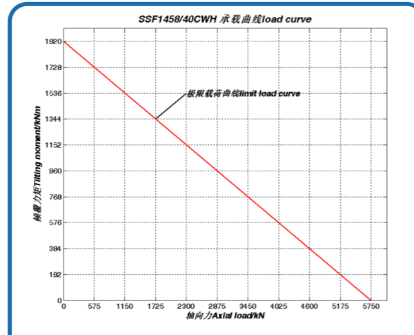
序号 46、SSF1458/40CWH 承载曲线
