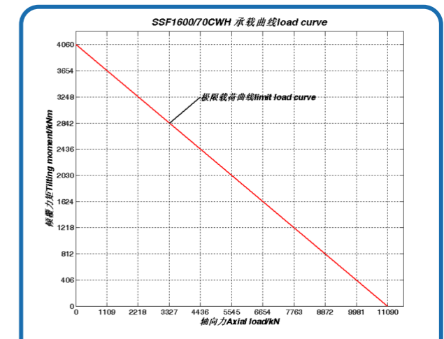
序号 56、SSF1600/70CWH 承载曲线
