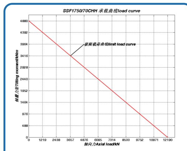
序号 62、SSF1750/70CHH 承载曲线
