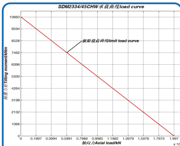
序号 21、SDM2334/45CHW 承载曲线
