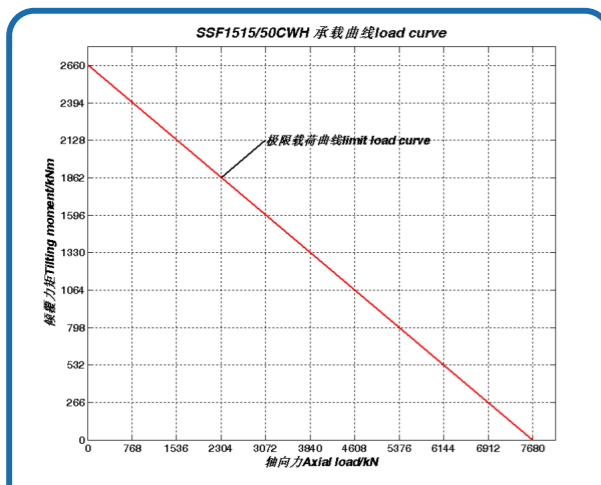
序号 49、SSF1515/50CWH 承载曲线
