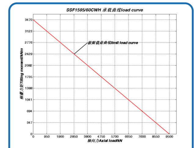
序号 54、SSF1595/60CWH 承载曲线
