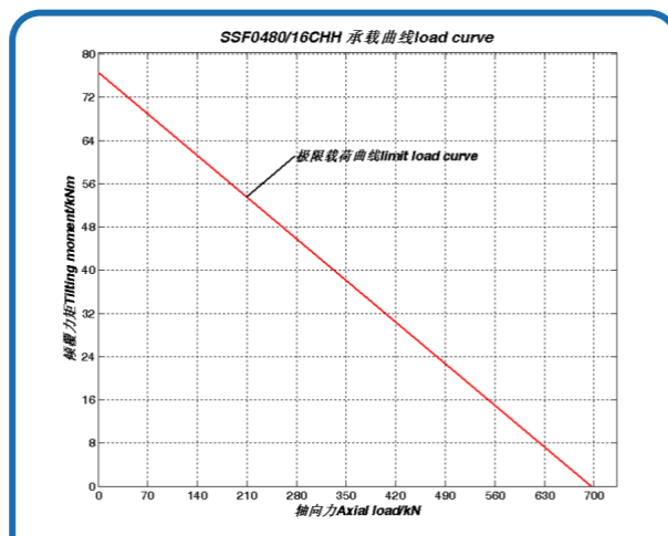
序号 2、SSF0480/16CHH 承载曲线
