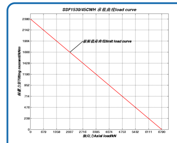
序号 53、SSF1530/45CWH 承载曲线
