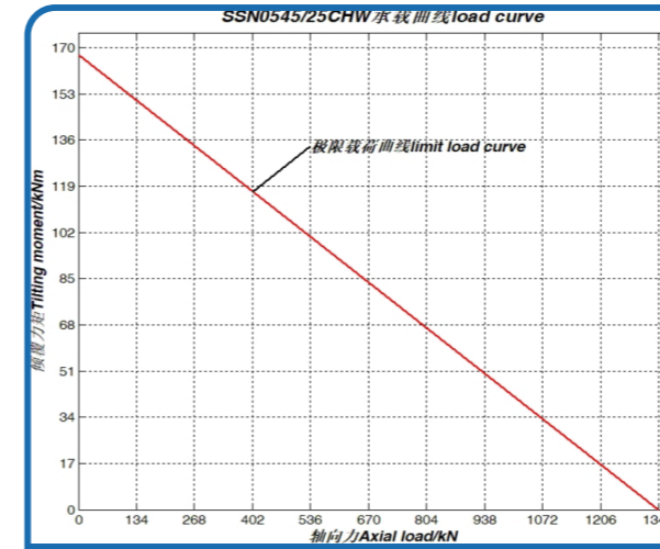
序号 7、SSN0545/25CHW 承载曲线
