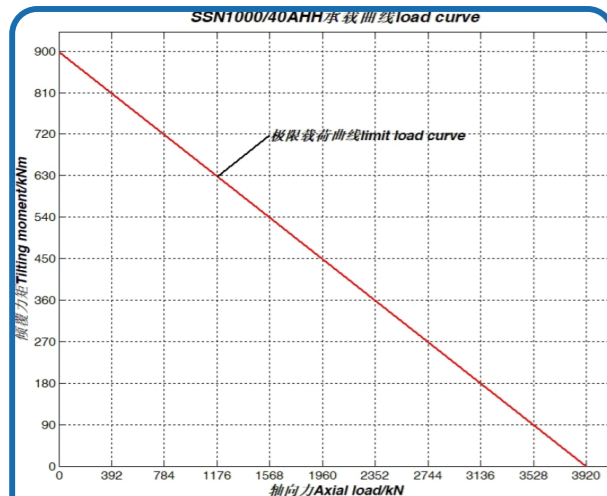
序号 13、SSN1000/40AHH 承载曲线
