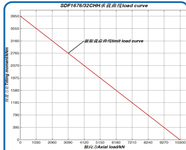
序号 10、SDF1676/32CHH 承载曲线
