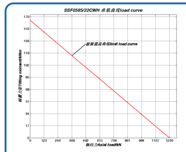
序号 5、SSF0585/22CWH 承载曲线
