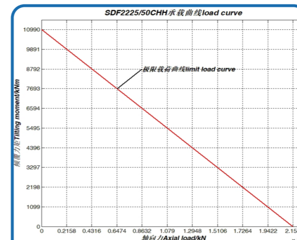
序号 19、SDF2225/50CHH 承载曲线
