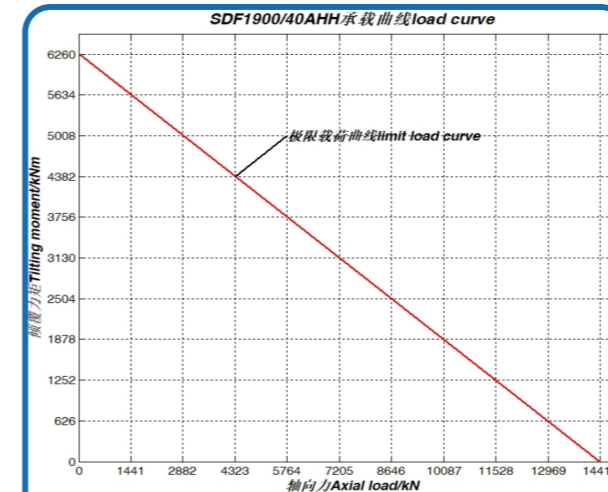
序号 15、SDF1900/40AHH 承载曲线
