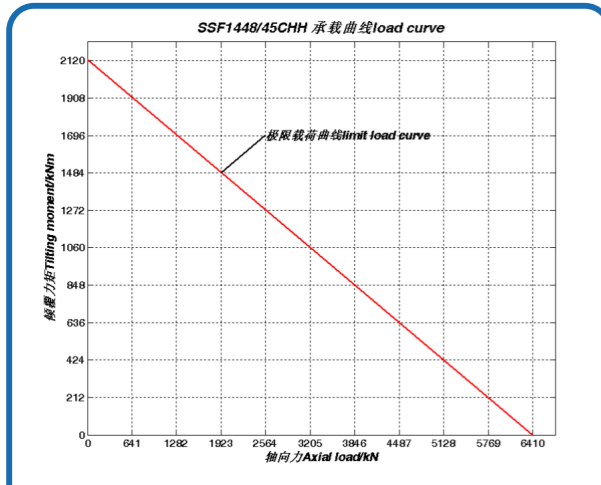
序号 45、SSF1448/45CHH 承载曲线
