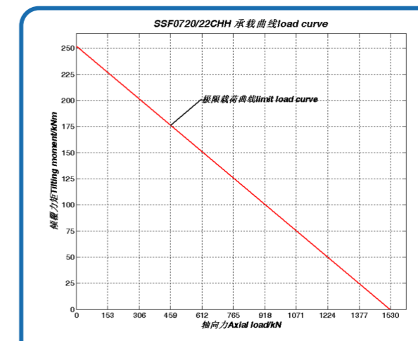
序号 8、SSF0720/22CHH 承载曲线
