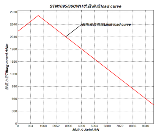
序号 5、STN1095/36CWH 承载曲线
