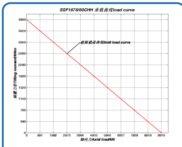
序号 59、SSF1676/60CHH 承载曲线
