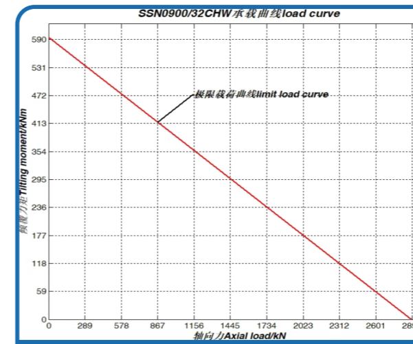
序号 11、SSN0900/32CHW 承载曲线
