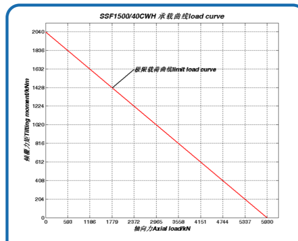
序号 48、SSF1500/40CWH 承载曲线
