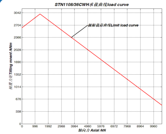
序号 8、STN1108/36CWH 承载曲线
