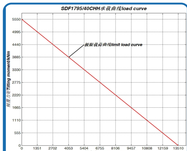
序号 13、SDF1795/40CHH 承载曲线
