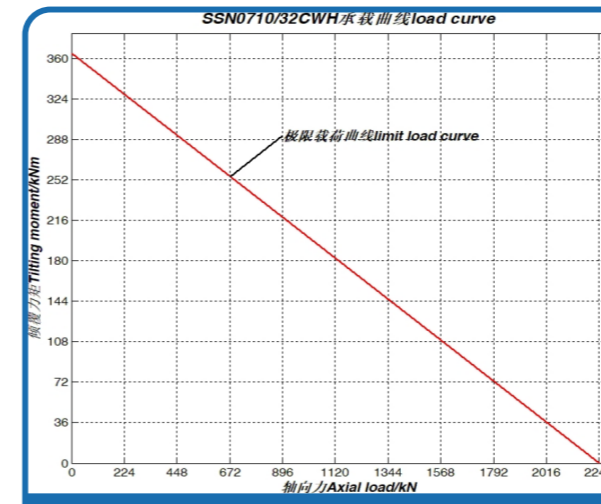
序号 9、SSN0710/32CWH 承载曲线
