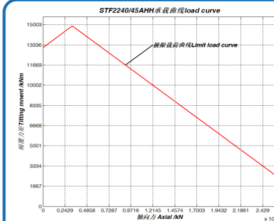
序号 6、STF2240/45AHH 承载曲线
