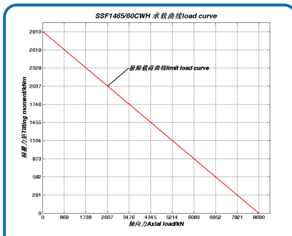
序号 47、SSF1465/60CWH 承载曲线
