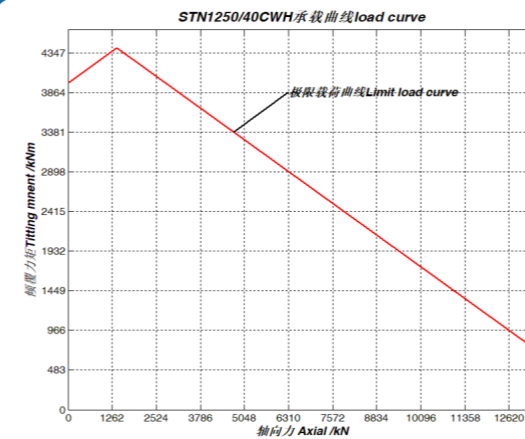
序号 9、STN1250/40CWH 承载曲线
