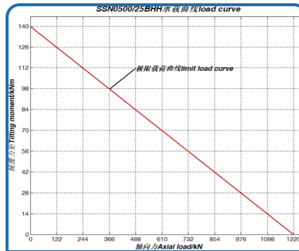
序号 4、SSN0500/25BHH II 承载曲线
