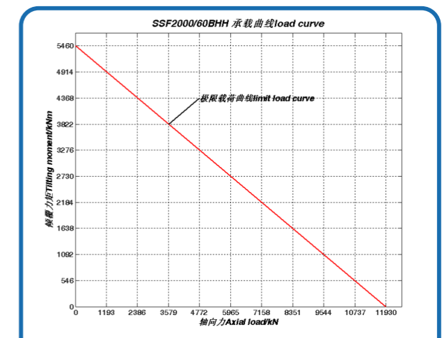
序号 66、SSF2000/60BHH 承载曲线
