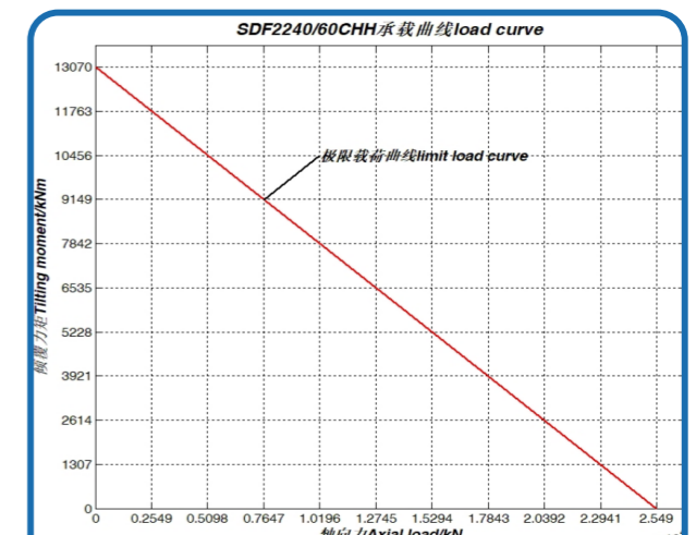
序号 20、SDF2240/60CHH 承载曲线
