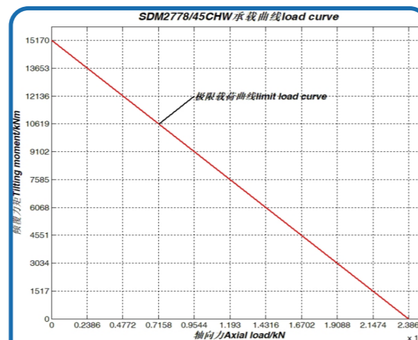
序号 24、SDM2778/45CHW 承载曲线
