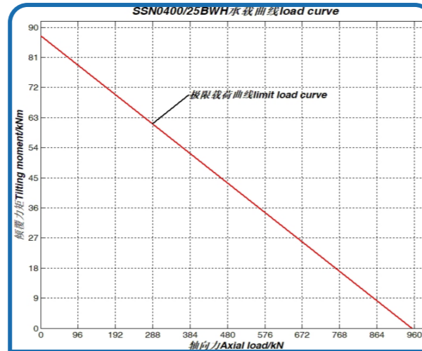
序号 2、SSN0400/25BWH 承载曲线
