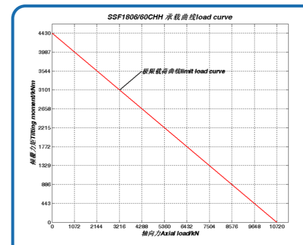
序号 65、SSF1806/60CHH 承载曲线
