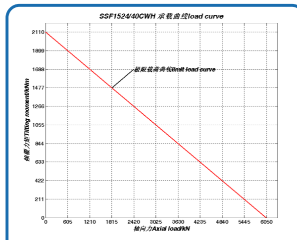
序号 50、SSF1524/40CWH 承载曲线
