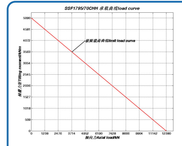
序号 63、SSF1795/70CHH 承载曲线
