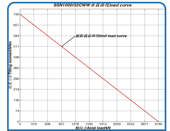
序号 12、SSN1000/32CWW 承载曲线
