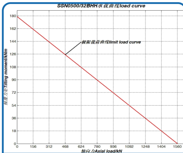
序号 5、SSN0500/32BHH 承载曲线
