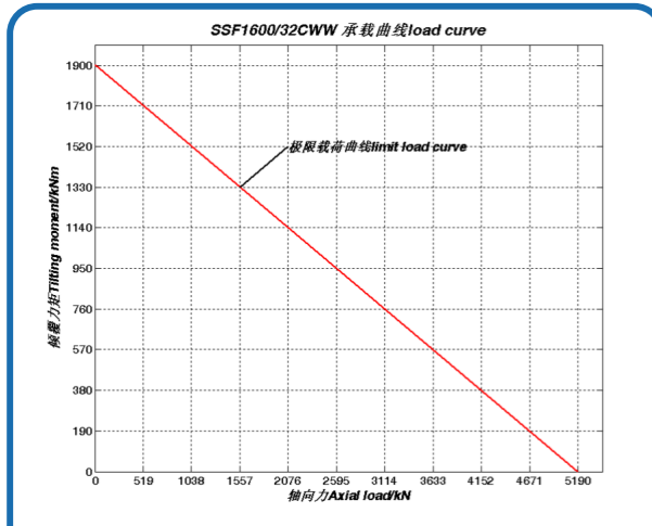
序号 57、SSF1600/32CWW 承载曲线
