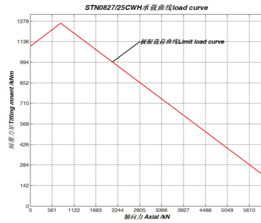
序号 2、STN0827/25CWH 承载曲线
