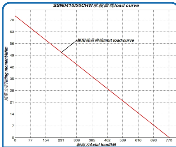
序号 3、SSN0410/20CHW 承载曲线
