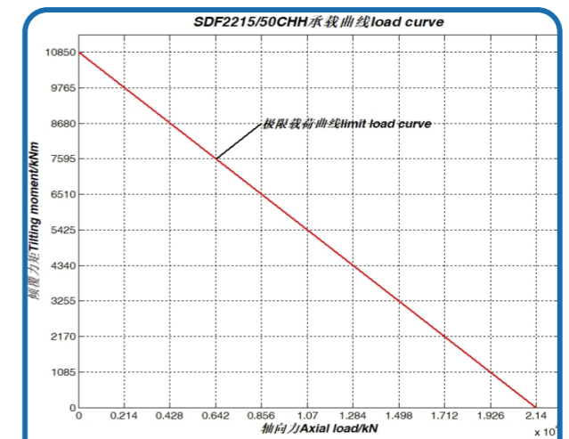
序号 18、SDF2215/50CHH 承载曲线
