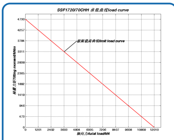
序号 61、SSF1720/70CHH 承载曲线
