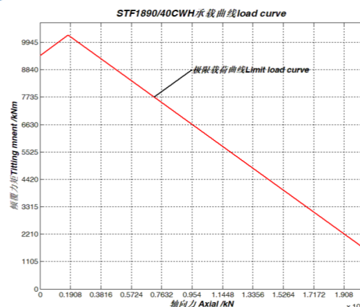
序号 3、STF1890/40CWH 承载曲线
