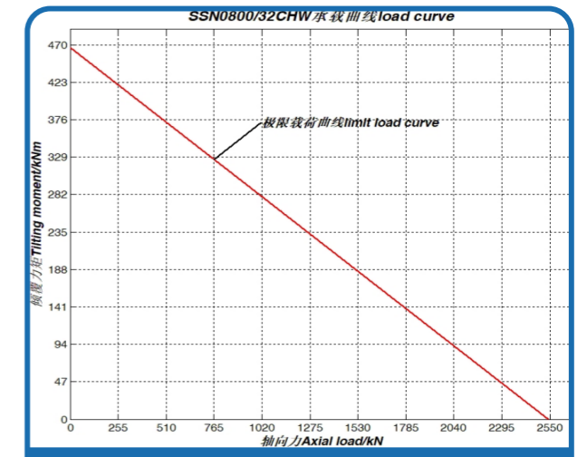
序号 10、SSN0800/32CHW 承载曲线
