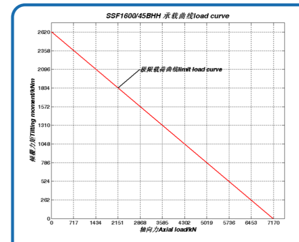
序号 55、SSF1600/45BHH 承载曲线
