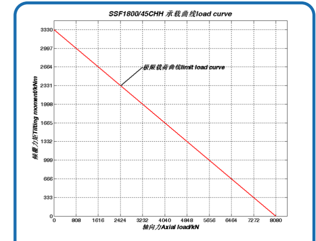
序号 64、SSF1800/45CHH 承载曲线
