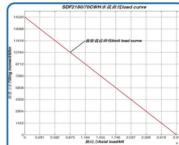
序号 17、SDF2180/70CWH 承载曲线
