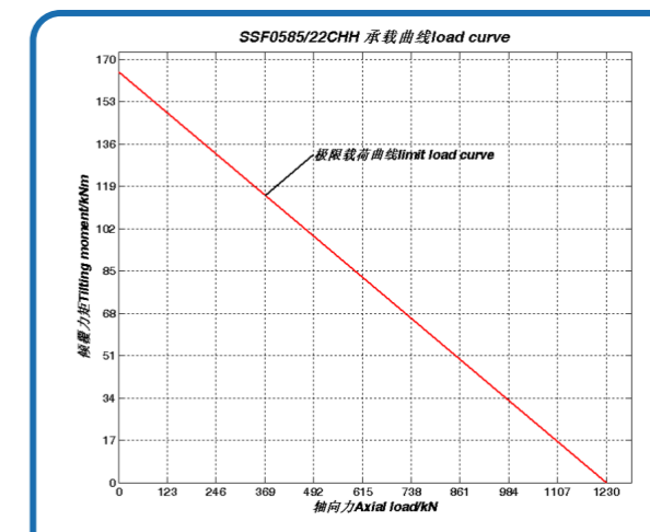
序号 4、SSF0585/22CHH 承载曲线
