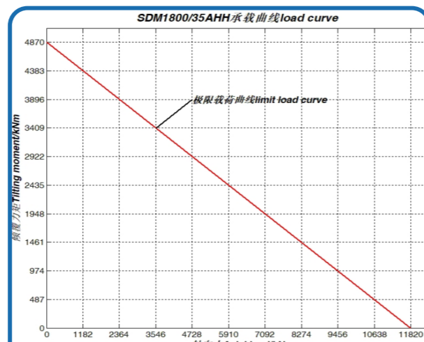
序号 14、SDM1800/35AHH 承载曲线
