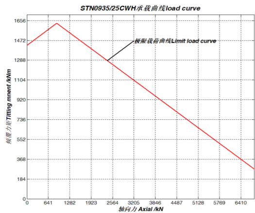
序号 3、STN0935/25CWH 承载曲线
