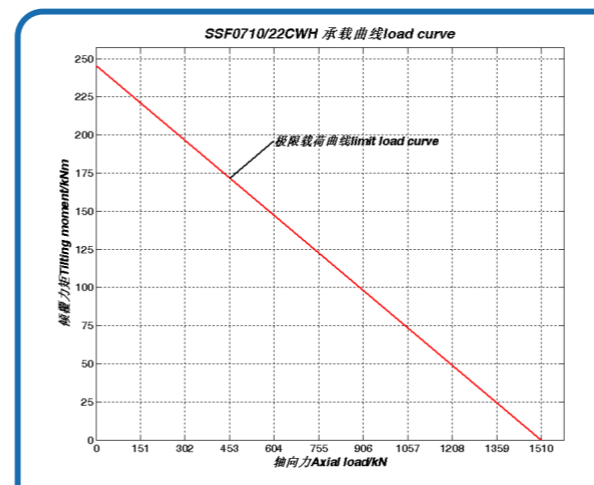
序号 7、SSF0710/22CWH 承载曲线
