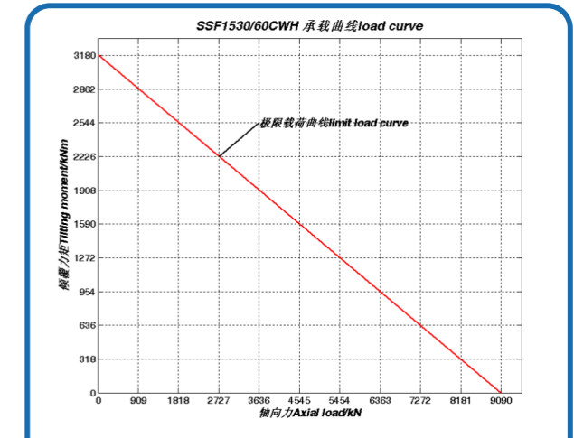
序号 52、SSF1530/60CWH 承载曲线
