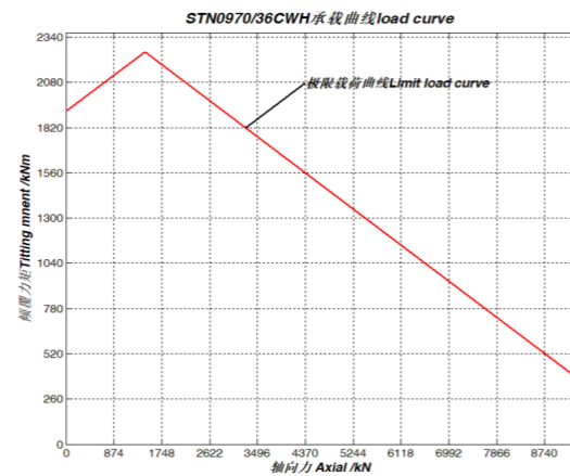
序号 4、STN0970/36CWH 承载曲线
