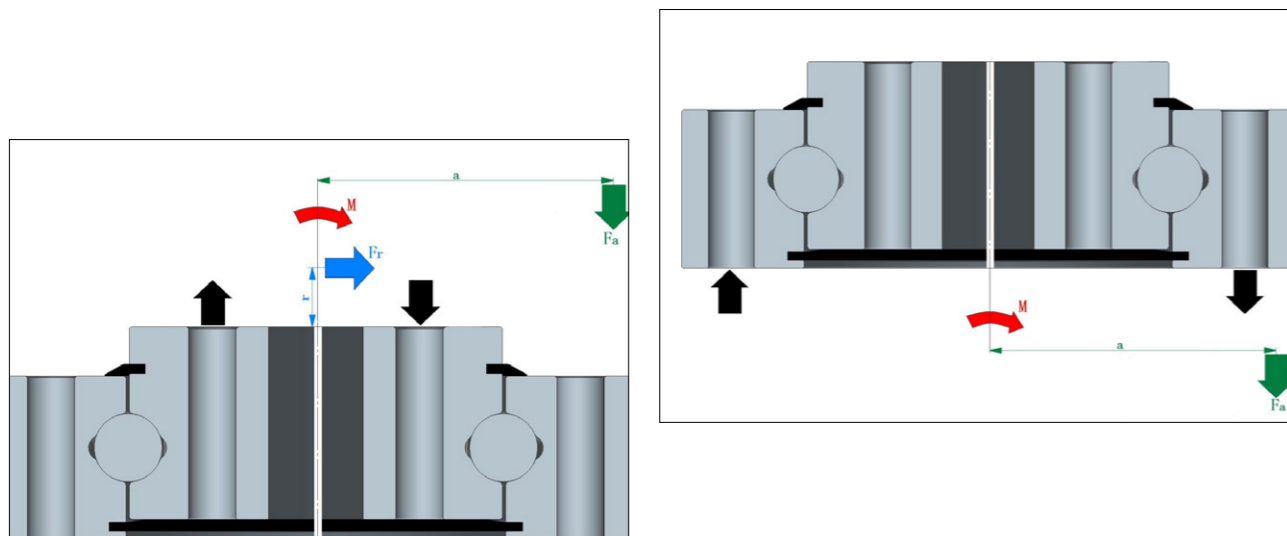
座式安装和悬挂式安装
