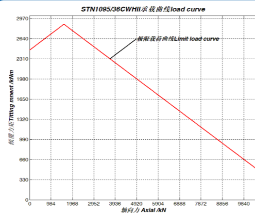
序号 6、STN1095/36CWH 承载曲线
