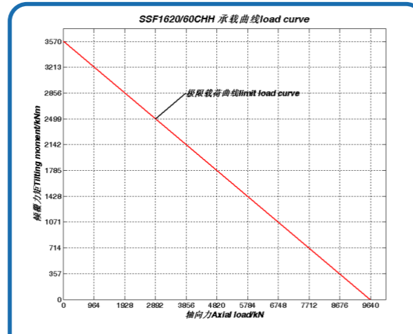
序号 58、SSf1620/60CHH 承载曲线
