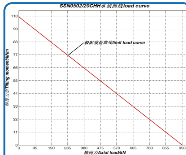
序号 6、SSN0502/20CHH 承载曲线
