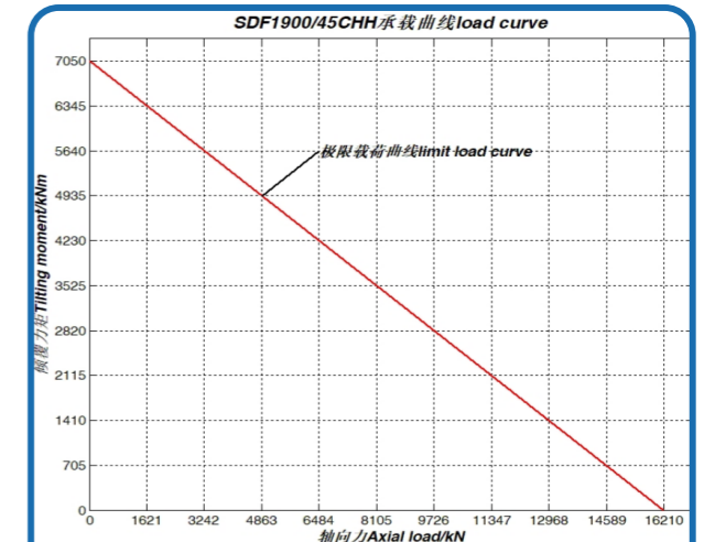
序号 16、SDF1900/45CHH 承载曲线
