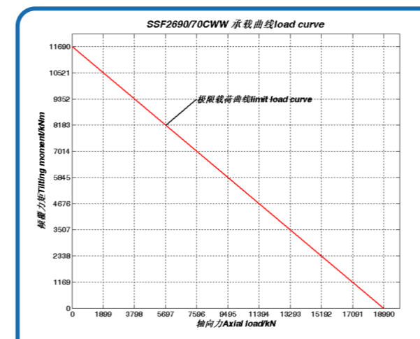
序号 67、SSF2690/70CWW 承载曲线
