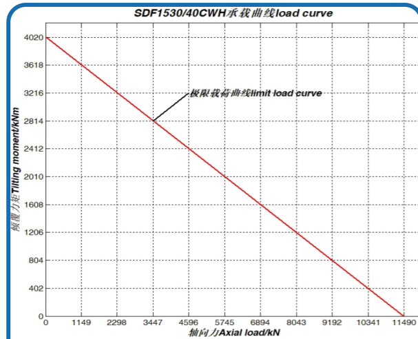
序号 9、SDF1530/40CWH 承载曲线
