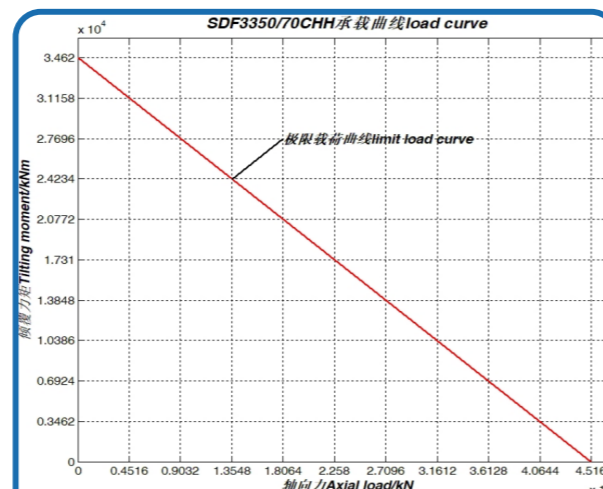
序号 26、SDF3350/70CHH 承载曲线
