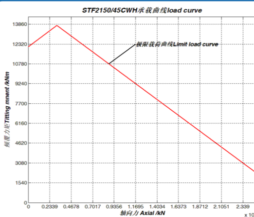
序号 5、STF2150/45CWH 承载曲线
