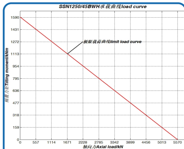
序号 15、SSN1250/45BWH 承载曲线
